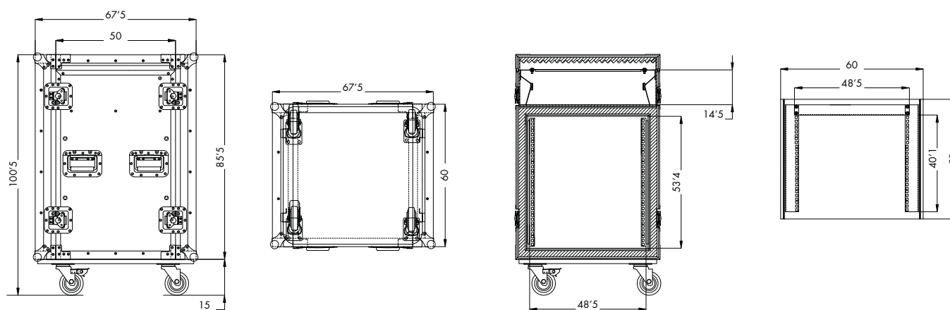
FRM-130
